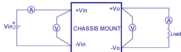
CQB150-300SXX-CMFC(D) Series Test Setup
